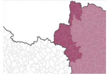
Radongebiete im Bezirk Gmünd ■ Radonvorsorge- und Radonschutzgebiet ■ Radonvorsorgegebiet, kein Radonschutzgebiet ■ kein Radonvorsorgegebiet, kein Radonschutzgebiet
